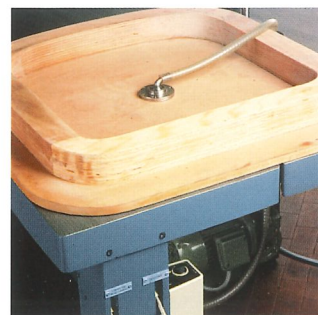
Vakuum-Saug-Spannanlage
