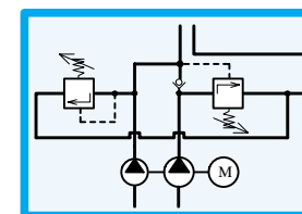
Pompa doppia con valvola disgiuntrice Two stage pump with pressure relief valve doppelte Pumpe mit Druckentlastungs-Ventil
