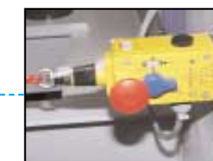
Fune più interruttore di sicurezza Perimeter E-stop System Sicherheits-Reißleine mit Schalter
